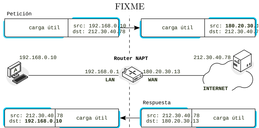
FIGURA 11.5: Ejemplo de SNAT
