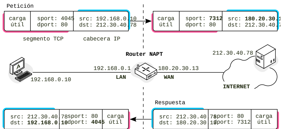
FIGURA 11.7: Ejemplo de NAT con puertos sintéticos
