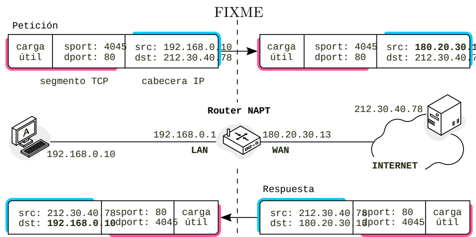
FIGURA 11.6: Ejemplo de NAT
